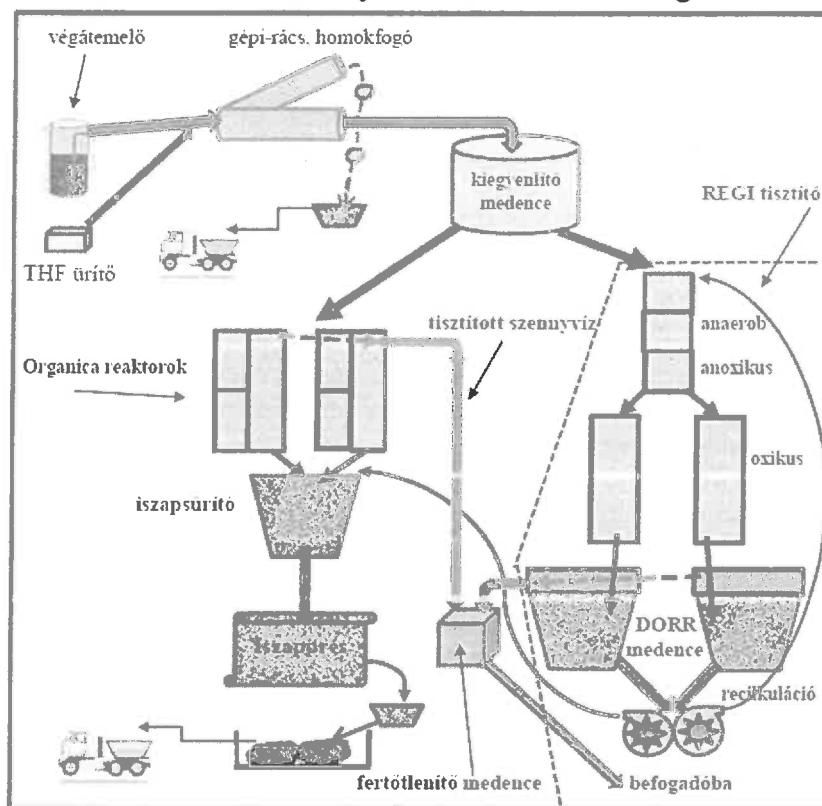
Szennyvíztisztítási technológia folyamatábrája
